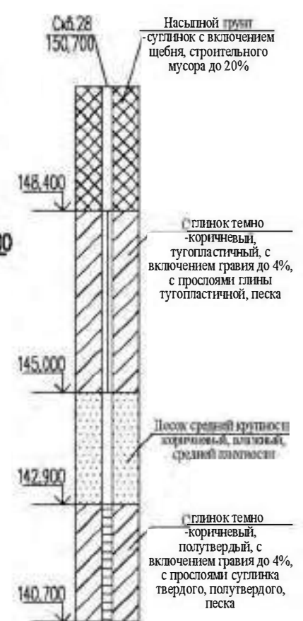
Рис. 62. Обеспечение сохранности ВОАН "Культурный слой села Дивеево". Нижегородская область. 2026 г. Продольный профиль сети.
